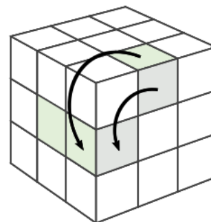
(B2) O^{-1}L^{-1}OLOVO^{-1}V^{-1}
