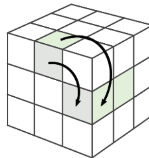
(B1) ORO^{-1}R^{-1}O^{-1}V^{-1}OV
